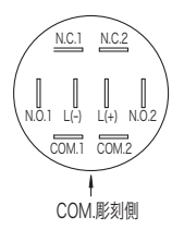
端子番号図
