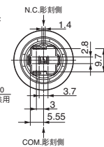
単極双投
