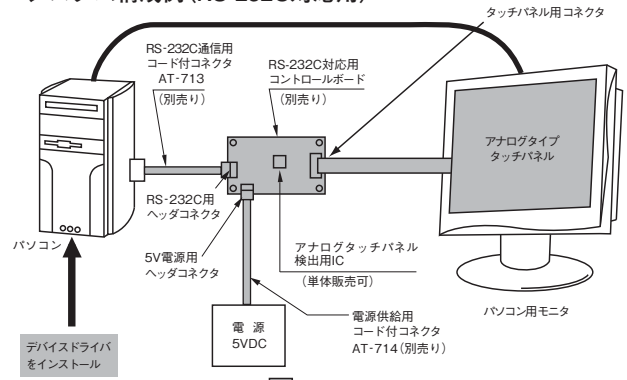
システム構成例 (RS-232C対応用)
